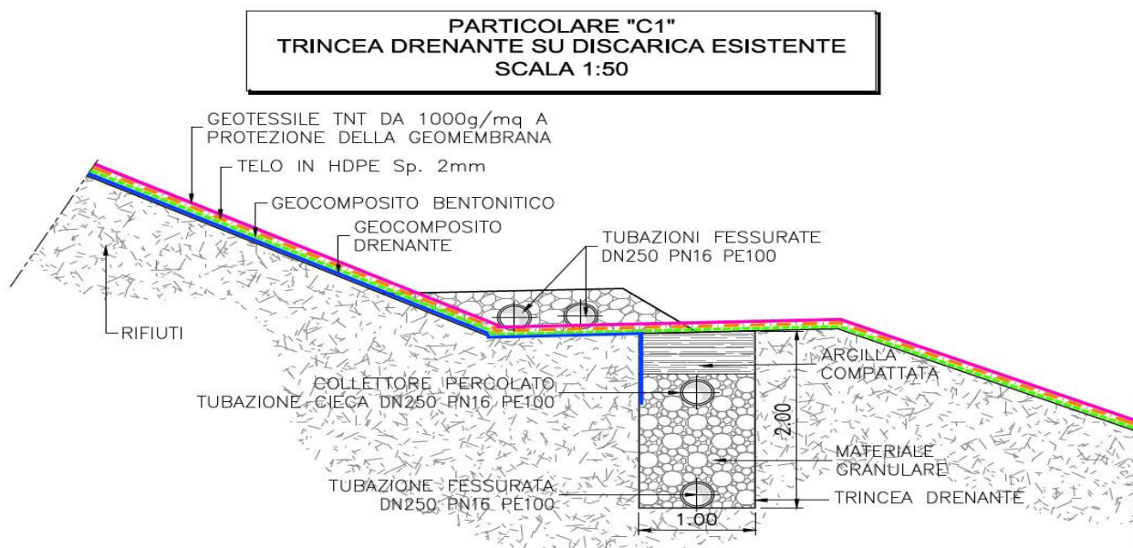
Figura 10 - Sezione del pacchetto del fondo discarica
