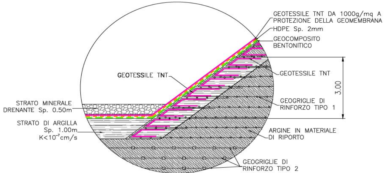
Figura 11 - Particolare "A2" – Barriera di protezione sul fondo
