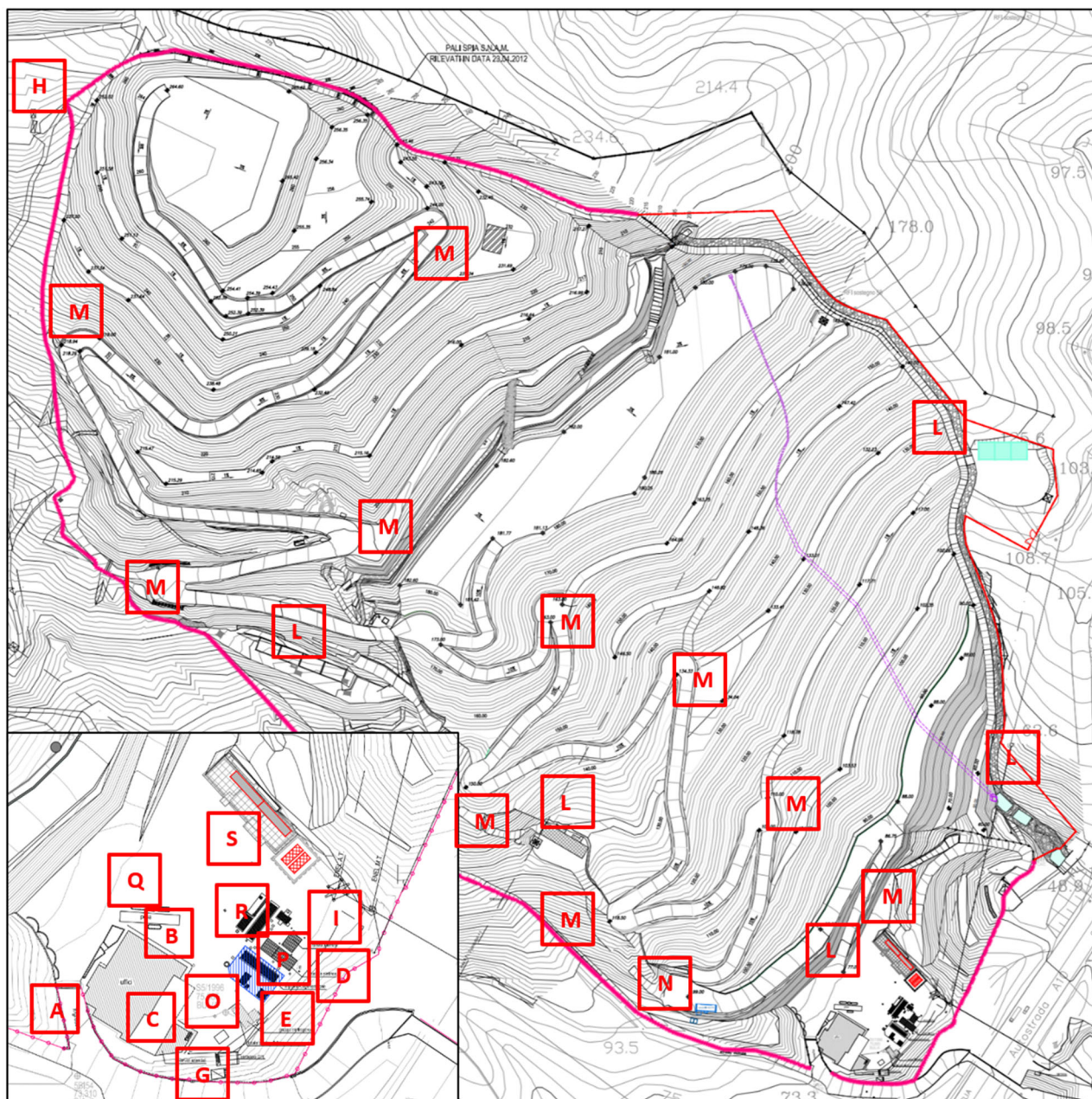
Figura 2 – Impianto di Bossarino – Planimetria allo stato attuale
