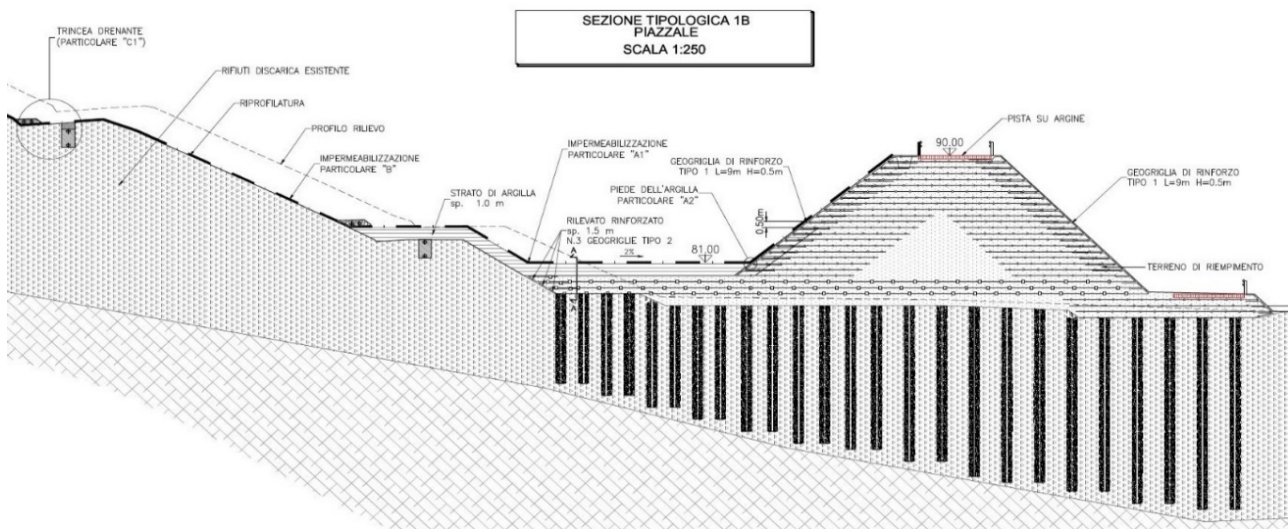
Figura 12 – Sezione tipologica piazzale
